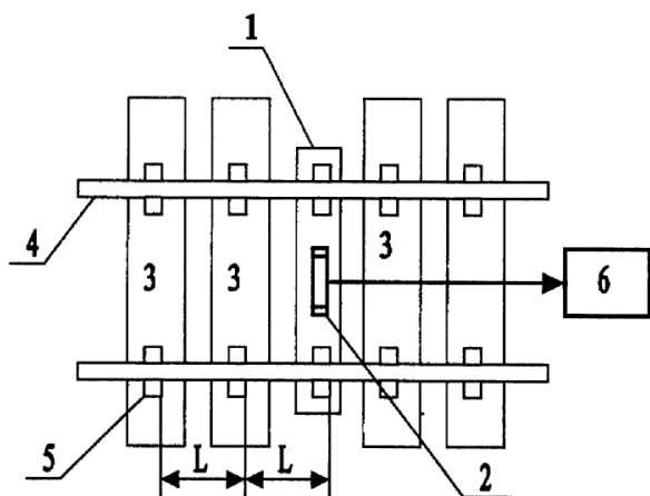
Рисунок 1 – Вагометричний пристрій:
