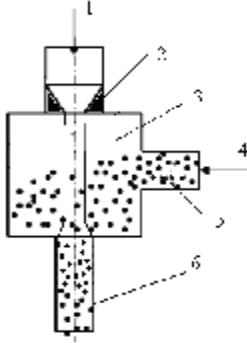
Рис. 1. Схема утворення гідроабразивного струменя
