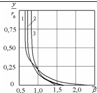
Рис. 4. Залежність концентрації абразивних частинок в перетині X=5 від кута конусності змішувальної камери: 1 – \alpha_k = 60^\circ ; 2 – \alpha_k = 45^\circ ; 3 – \alpha_k = 30^\circ
