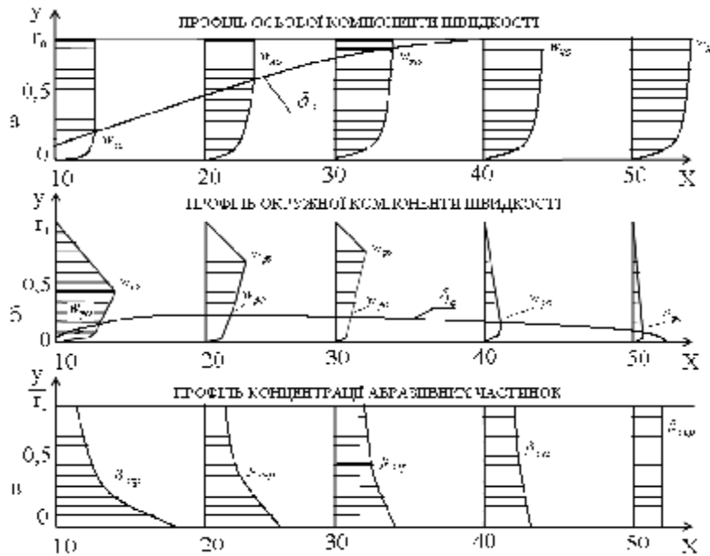
Рис. 2. Розподіл швидкостей двофазного потоку та концентрації абразиву в перетинах по довжині каналу: а – профіль осьовий компоненти швидкості, б – профіль окружної компоненти швидкості, в – профіль концентрації
