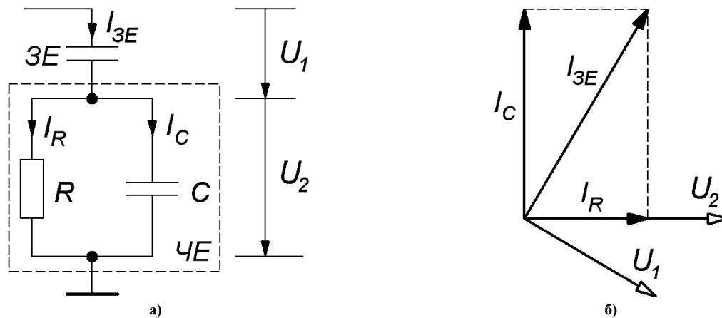
Рис. 3. Електрична еквівалентна схема вимірювального перетворювача (ВП) ємнісного вологоміра (а) та векторна діаграма напруг і струмів вимірювального перетворювача вологості (б)
