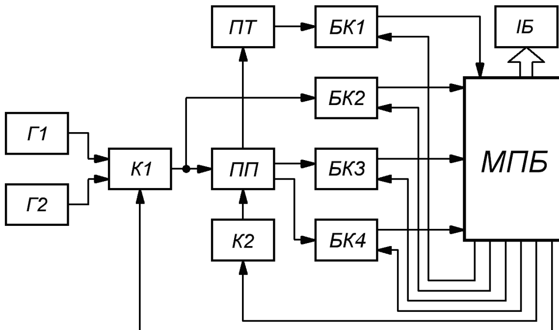
Рис. 4. Структурна схема засобу контролю вологості слабо зволоженого зерна
