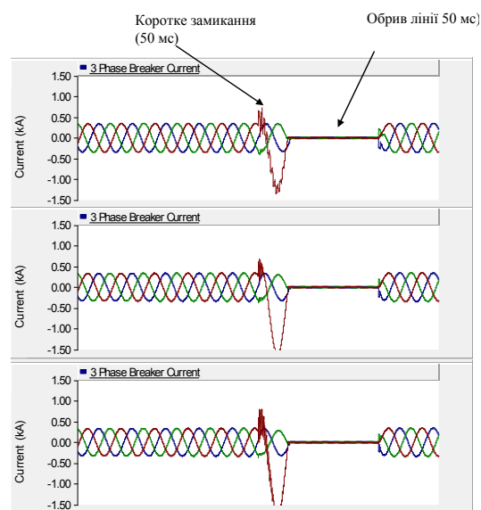
Рис. 5. Зміна струму через розривач на навантаження
