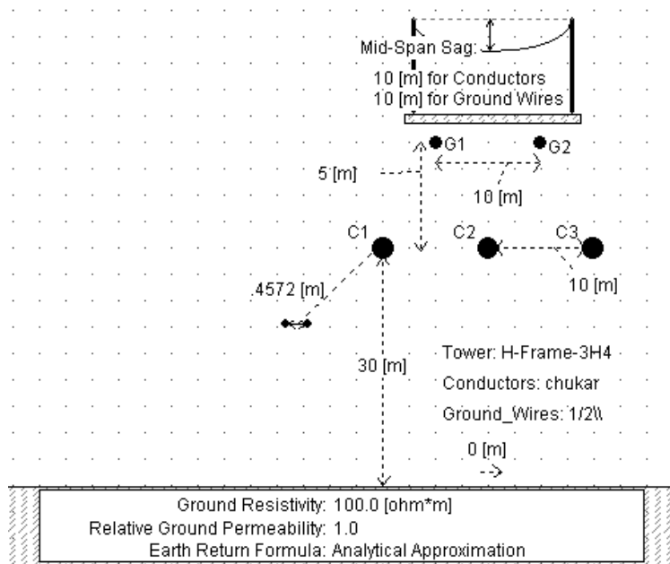
Рис. 2. Бергеронова модель досліджуваної лінії та параметри цієї моделі
