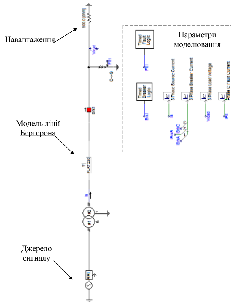
Рис. 1. Структурна схема лінії для моделювання
