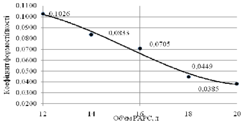
Рис. 2. Залежність коефіцієнта формостійкості від об'єму РАРС, при дослідженні пальтової тканини 3506
