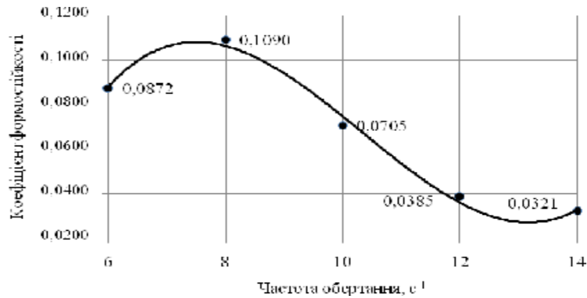
Рис. 1. Залежність коефіцієнта формостійкості від частоти обертання барабана, при дослідженні пальтової тканини 3506
