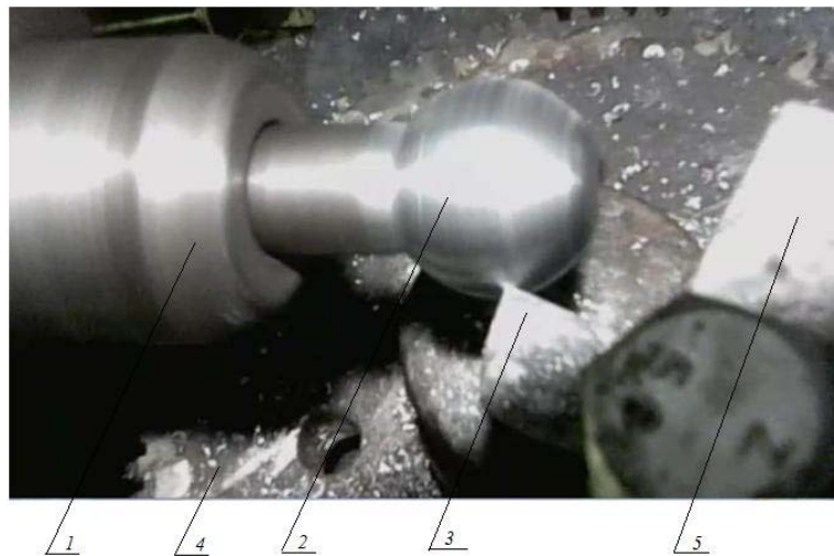
Рис. 9. Фрагмент процесу токарної обробки сфери кульового пальця з використанням поворотного пристрою: 1 – спеціальна оправка; 2 – заготовка; 3 – різець; 4 – поворотний стіл; 5 – різетримач
