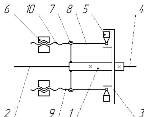
Рис. 1. Кінематична схема відцентрової фрикційної муфти з регульованим крутним моментом
