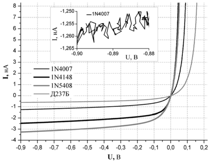
Рис. 9. ВАХ кремнієвих діодів при малих струмах
