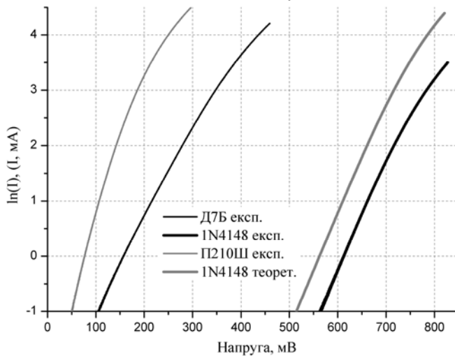
Рис. 8. Залежності \ln(I) , ( I , мА) від напруги на діодах при прямому включенні
