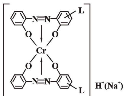
Рис. 3. Хімічна формула третьої групи металокомплексних барвників 1:2
