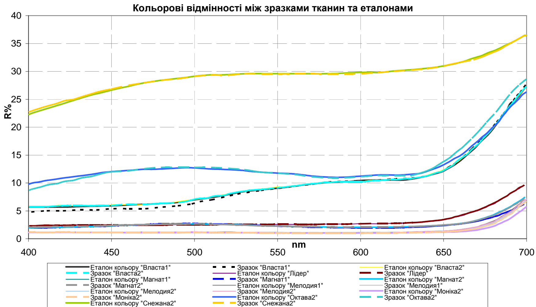
Рис. 4. Результати порівняння пофарбування зразків тканин зі спеціальним обробленням зі зразками-еталонами цих тканин, одержані на спектрофотометрі
