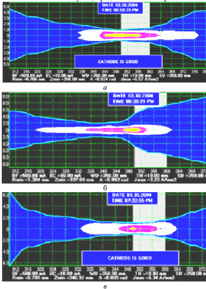
Рис. 3. Модели восстановления профилей плотности тока в пучке: а – пушка 1; б – пушка 2; в – пушка 3
