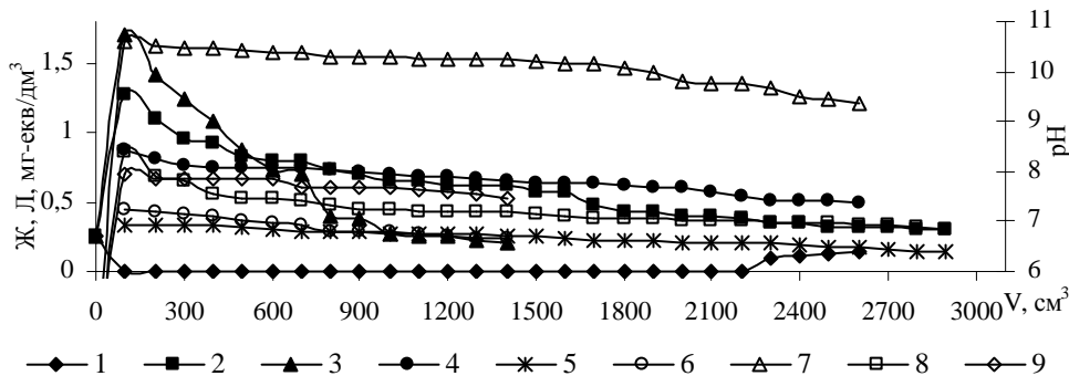
Рис. 4. Зміна жорсткості (1; 2; 3), лужності (4; 5; 6), та рН (7; 8; 9) перміату ( Ж = 0,26 мг-екв/дм 3 , K = 0,70 мг-екв/дм 3 , pH = 3,94 ) в залежності від пропущеного об’єму через катіоніт DOWEX MAC-3 в K^+ (1; 3; 7), Ca^{2+} (2; 5; 8), Mg^{2+} (3; 6; 9) формі
