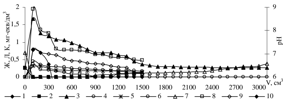
Рис. 3. Залежність жорсткості (1; 2; 3), лужності (4; 5; 6), кислотності (7) та рН (8; 9; 10) розчину від пропущеного об'єму перміату ( Ж = 0,26 \text{ мг-екв/дм}^3, К = 0,70 \text{ мг-екв/дм}^3, \text{ рН} = 3,94 ) через іоніт КУ-2-8 в Na^+ (1; 4; 8), K^+ (2; 5; 9), Ca^{2+} (3; 6; 7; 10) формі
