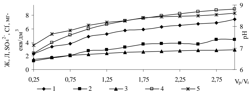
Рис. 2. Вплив співвідношення об'ємів вихідного модельного розчину ( Ж = 9,35 мг-екв/дм 3 , Л = 5,80 мг-екв/дм 3 , рН = 8,96 ) та перміату ( Ж = 0,26 мг-екв/дм 3 , К = 0,70 мг-екв/дм 3 , рН = 3,94 ;
