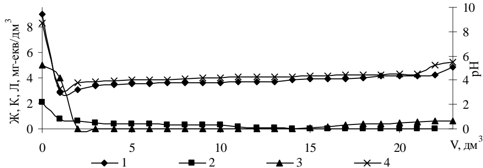
Рис. 1. Залежність жорсткості (1), кислотності (2), лужності (3) та рН (4) модельного розчину ( Ж = 9,0 мг-екв/дм 3 , Л = 5,0 мг-екв/дм 3 , C(SO_4^{2-}) = 576,0 мг/дм 3 , C(Cl) = 126,0 мг/дм 3 ) від пропущеного об'єму через іоніт DOWEX MAC-3 в кислій формі ( V_i = 50 см 3 ) ( OC_1 = 2,489 г-екв/дм 3 , OC_3 = 2,362 г-екв/дм 3 )
