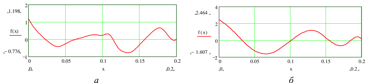
Рис. 7. Кореляційні функції круглограм оброблених поверхонь зразків-виробів, визначені засобами пакета MathCAD: а – \delta_0=30 мкм; б – \delta_0=40 мкм
