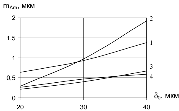
Рис. 5. Математичне сподівання амплітуд суттєвих гармонік m_{Am} поверхонь партії зразків-виробів у функції зазору \delta_0 регульованих шпindelних ГСО (номер кривої відповідає номеру гармоніки спектра)
