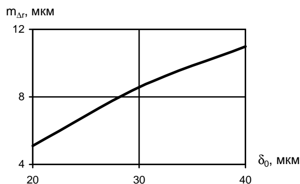
Рис. 2. Математичне сподівання відхилень від круглості m_{\Delta r} поверхонь партії зразків-виробів у функції зазору \delta_0 регульованих шпиндельних ГСО
