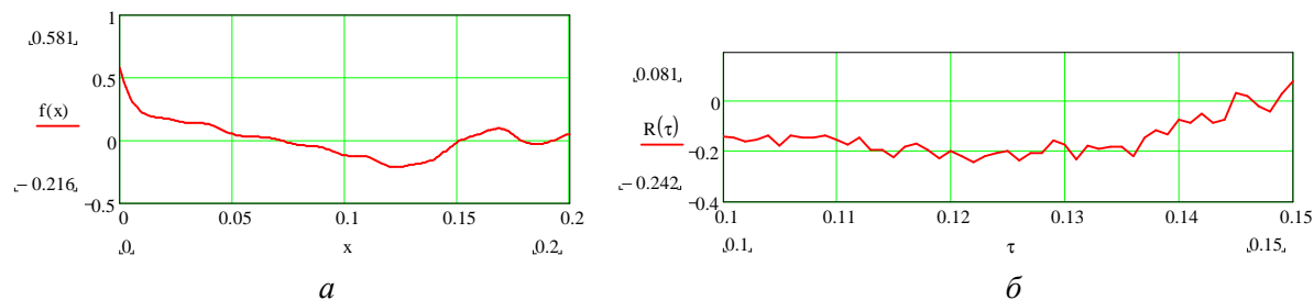
Рис. 6. Кореляційна функція круглограми обробленої поверхні при \delta_0=20 мкм у регульованих ГСО шпинделя, визначена засобами пакета MathCAD (графіки на рис. а, б визначають кореляційну функцію в різних масштабах по осі абсцис)
