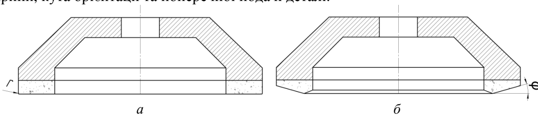
Рис. 2. Профіль шліфувального круга: а – нового, б – зношеного
