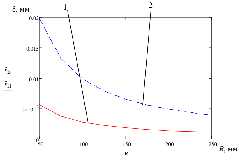
Рис. 5. Графік залежності \delta від R
