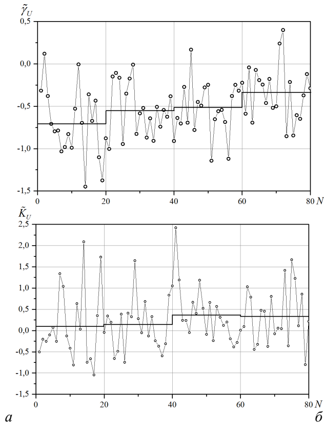
Рис. 2. Закономірності зміни коефіцієнта асиметрії \tilde{\gamma}_U (а) та коефіцієнта ексцесу \tilde{K}_U (б) амплітуди результуючого сигналу акустичної емісії, який зареєстровано при різних швидкостях обертання вузла тертя із композиційних матеріалів
