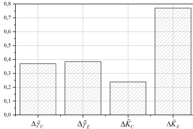
Рис. 5. Абсолютний приріст значень коефіцієнтів асиметрії та ексцесу амплітуди та енергії результуючих сигналів акустичної емісії, які формуються при третій поверхонь із композиційних матеріалів
