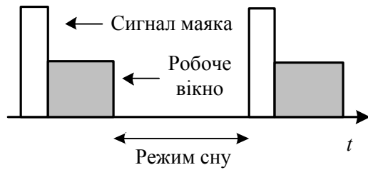
Рис. 2. Структура часових пакетів мережі Mesh Lite
