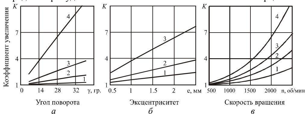
Рис. 2. Зависимость коэффициента увеличения силы отрыва капли от различных параметров: a - l_1 = l_2 = 30 мм; e = 1,0 мм; n = 500, 1000, 1500, 2500 об/мин, графики 1, 2, 3, 4 соответственно; b - l_1 = l_2 = 30 мм; n = 1500 об/мин, \gamma = 10, 20, 50^\circ , графики 1, 2, 3 соответственно; v - l_1 = l_2 = 30 мм; e = 1,0 мм; \gamma = 10, 20, 30, 50^\circ , графики 1, 2, 3, 4 соответственно
