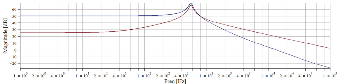
Рис. 5. Діаграма Бode на основі динамічної моделі
