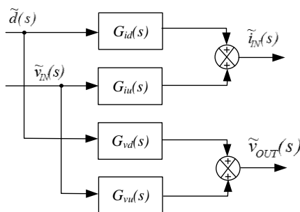
Рис. 4. Малосигнальна модель однофазного трирівневого КІІ з фіксованою нейтральною точкою
