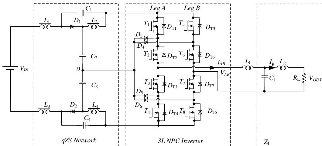
Рис. 1. Схема трирівневого однофазного КІП
