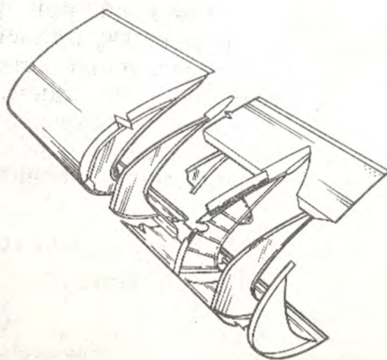
Рис. 3. Конструкція передкрилка з боропластика літака С-5А
