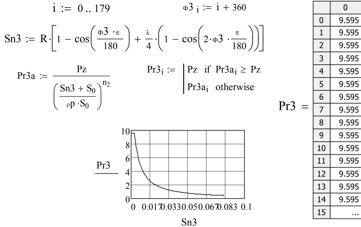
Рис. 3. Значення показників і параметрів при такті розширення двигуна
