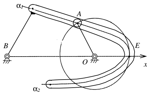
Рисунок 10 – Кулисный механизм с криволинейной кулисой, имеющей две ветви
