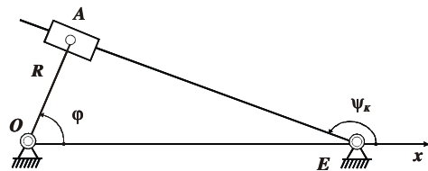
Рисунок 5 - Базовый механизм для кулисного механизма с криволинейным пазом, в котором выходное звено совершает качательное движение
