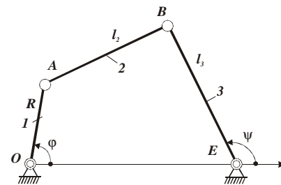
Рисунок 1 - ШЧ с выходным звеном коромыслом
