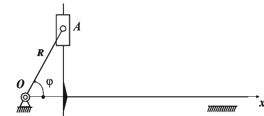
Рисунок 6 - Базовый механизм для кулисного механизма с криволинейным пазом, в котором выходное звено совершает поступательное движение
