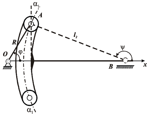
Рисунок 4 - Кулисный механизм с криволинейным пазом с поступательным движением выходного звена
