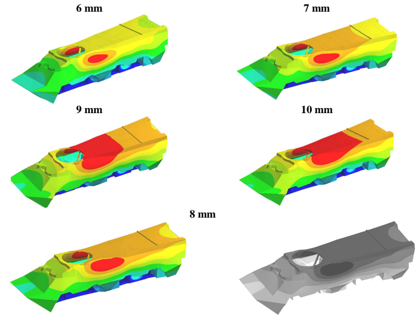
Рисунок 2 – Некоторые собственные формы колебаний для номинального (8 мм) распределения толщин и при варьировании толщин (1-я собственная частота)
