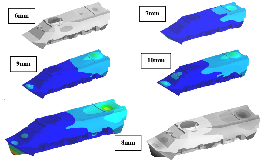
Рисунок 2 – Некоторые собственные формы колебаний для номинального (8 мм) распределения толщин и при варьировании толщин (4-я собственная частота)
