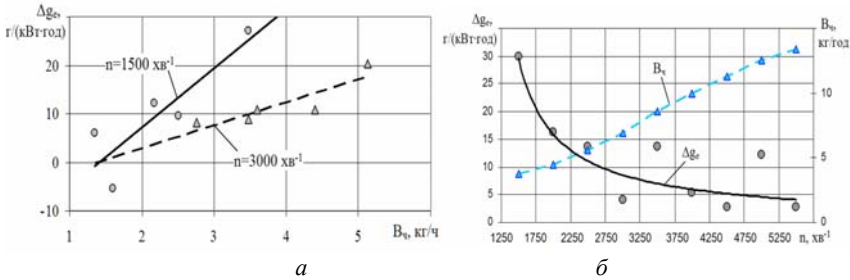
Рис. – Зменшення питомої ефективної витрати палива \Delta g_e двигуна 4C7,2/6,7 при введєнні корундового покриття донця поршня за навантажувальними a та зовнішньою швидкісною б характеристиками
