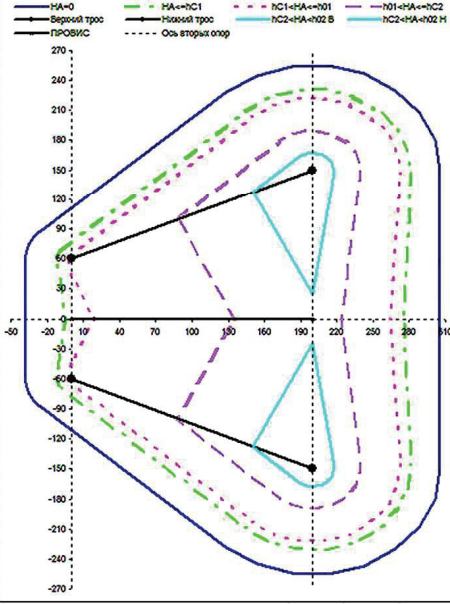
Рисунок 2 – Интерфейс программы расчета параметров зоны защиты двойного наклонного непараллельного тросового молниеотвода и построения границ зоны защиты ДННПТМО на заданных высотах анализа
