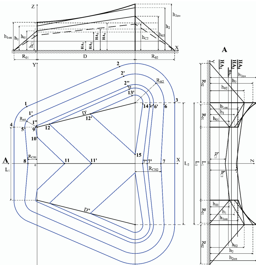
Рисунок 1 – Зона защиты наклонного непараллельного тросового молниеотвода и ее границы на пяти высотах анализа (НА1, НА2, НА3, НА4 и уровне грунта) при h_{10n} < h_{20n} :
