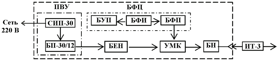
Рисунок 5 – Блок-схема генератора ИГЛА-МКУ-3-1 МГц:
