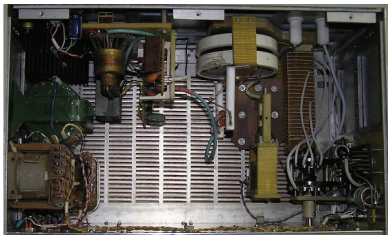
Рисунок 4 – Расположение элементов внутри корпуса генератора ИГЛА-МКУ-3-1 МГц
