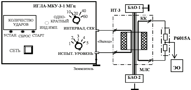
Рисунок 9 – Схема испытаний БАО:
