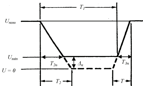
Рисунок 1 – Форма провалов напряжения для БАО с цифровыми схемами (КПЦС)
