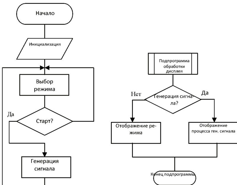
Рисунок 5 – Алгоритм работы программы СПЦС-А
