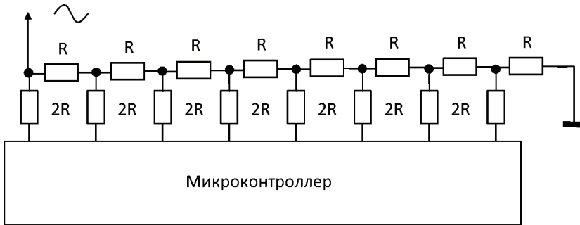
Рисунок 4 – Схема функциональная ЦАП - R 2R
