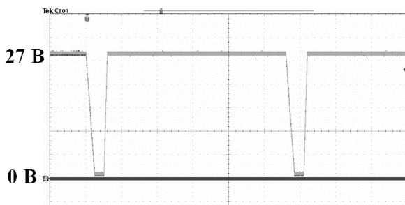
Рисунок 9 – Циклограмма испытательного напряжения вида КПЦС
