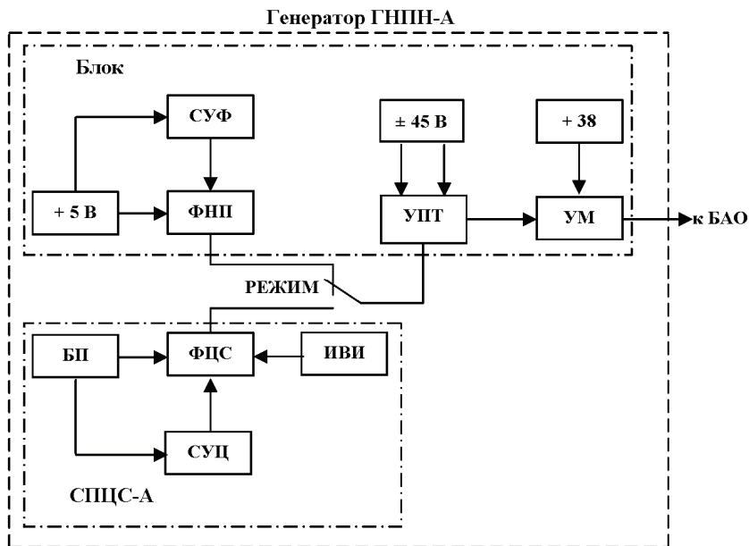
Рисунок 2 – Структурная схема генератора ГНПП-А:
