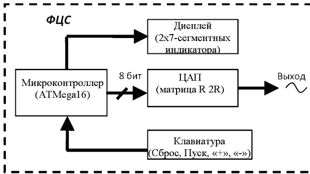
Рисунок 3 – Блок-схема ФЦС
