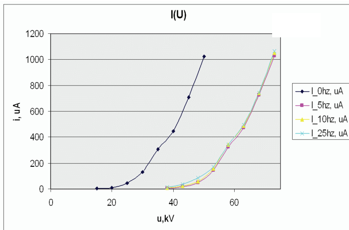
Рисунок 3 – ВАХ при различных частотах следования импульсов для положения 1 ( a ) и 5 ( б ) дополнительных коронирующих электродов
