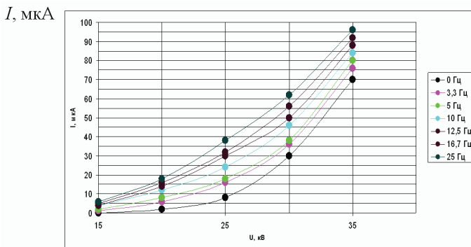
Рисунок 1 – ВАХ нагрузки без дополнительных коронирующих электродов для различных частот следования импульсов напряжения
