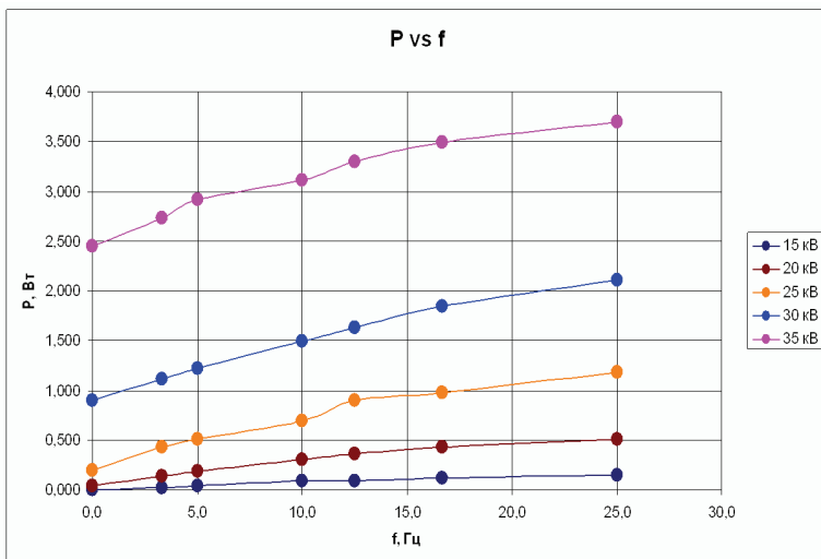
Рисунок 4 – Зависимость мощности отдаваемой в нагрузку комбинированной системой питания от частоты следования высоковольтных импульсов при различных напряжениях
