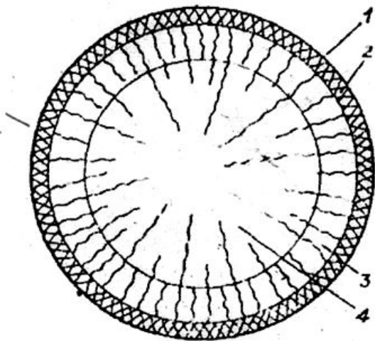
Рис. 3 – Модель дефектной структуры частицы, формирующейся в процессе механической обработки порошков: 1 – поверхностный слой, содержащий сорбированные газы; 2 – поверхностный, сильно разупорядоченный слой; 3 – приповерхностный пластически деформированный слой, содержащий микротрещины; 4 – слабо искаженное ядро частицы.
