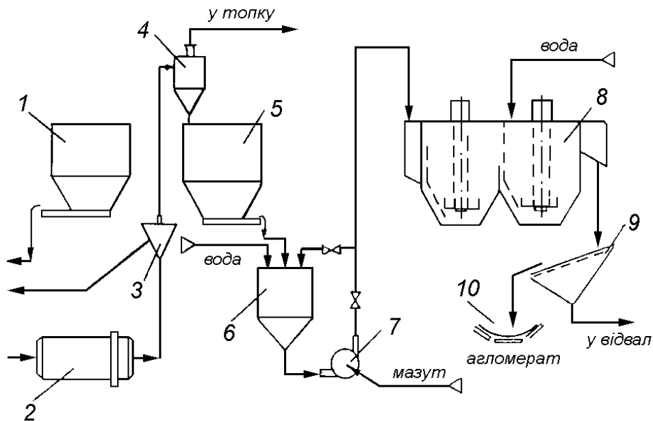
Рис.7. Пілотна установка масляної грануляції піловидного вугілля на Луганській ТЕС
