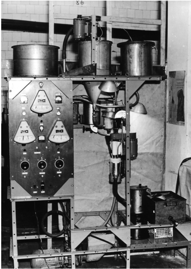
Рис.1. Стендова установка процесу селективної масляної агрегації на кафедрі „Збагачення корисних копалин” Донецького політехнічного інституту (1982-1986 р.р.).
