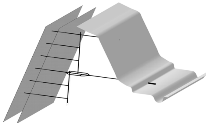
Рис. 3 Розкриття крутих пластів штольнями
