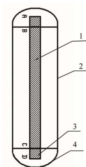
Рис. 1. Схема дії камуфлетного циліндричного заряду: 1 – заряд; 2 – контур порожнини; 3 – „ефективна” частина заряду; 4 – контур торцевої частини порожнини.
