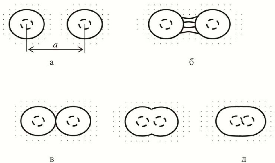
Рис. 2. Поперечні перерізи порожнин, утворених одночасним вибухом двох подовжених циліндричних зарядів в в'язучому ґрунті:
