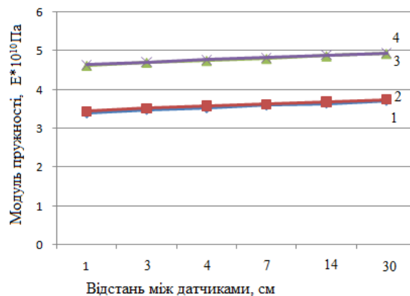
Рис.3. Для Покостівського граніту. Криві 1,2 - значення модуля пружності, E \cdot 10^{10} (Па) при вибуховому способі видобування блоків по горизонталі і по вертикалі відповідно, криві 3,4 - значення модуля пружності, E \cdot 10^{10} (Па) при способі видобування блоків із застосуванням алмазно-канатних пил, по горизонталі і по вертикалі відповідно.
