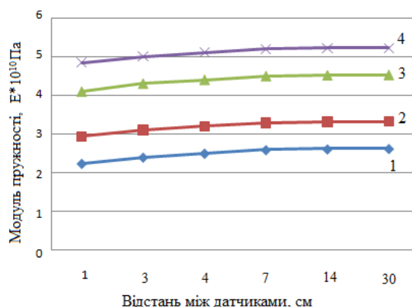
Рис.5. Для Корнинського граніту. Криві 1,2 - значення модуля пружності, E \cdot 10^{10} (Па) при вибуховому способі видобування блоків по горизонталі і по вертикалі відповідно, криві 3,4 - значення модуля пружності, E \cdot 10^{10} (Па) при способі видобування блоків із застосуванням алмазно-канатних пил, по горизонталі і по вертикалі відповідно.
