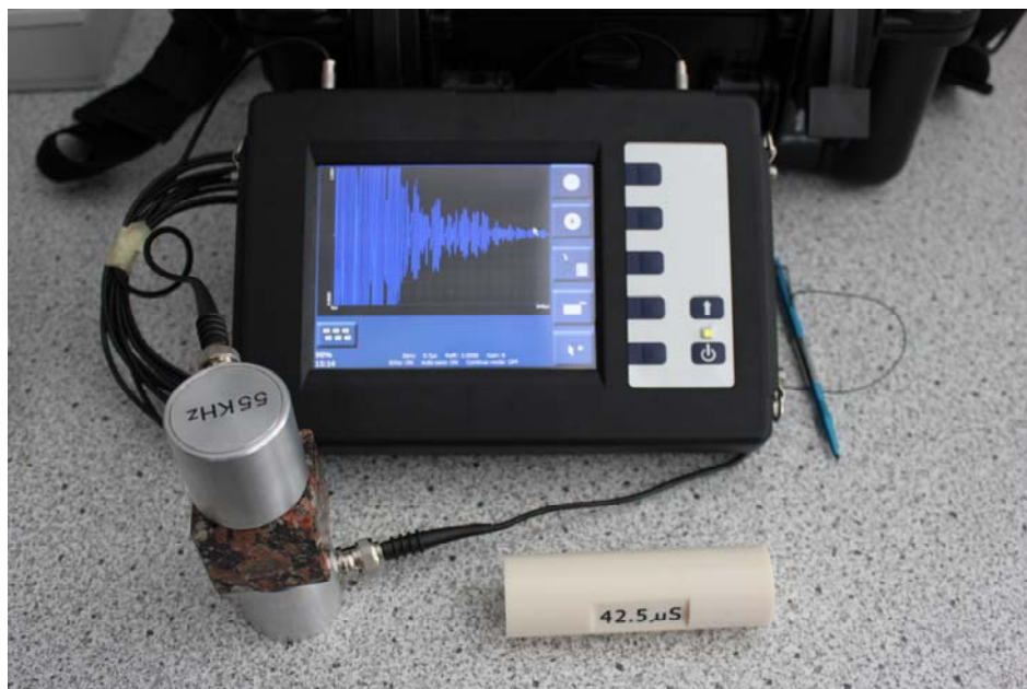
Рис.2. Ультразвуковий дефектоскоп італійської фірми MATEST модель C372N
