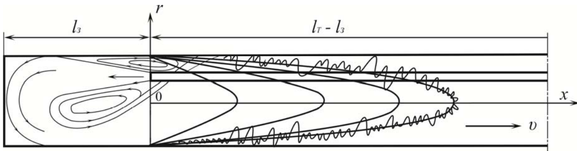
Рис. 1. Схема деформации и растяжения пылевого облака в тупиковой выработке при нестационарном процессе поступления пыли и нагнетательном способе проветривания.
