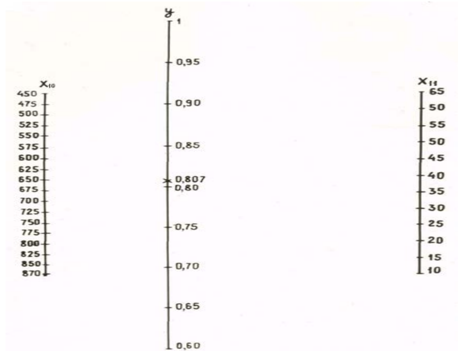
Рис. 3. Номограмма зависимости физиологического состояния ( y ) от средневзвешенной поверхностной плотности X_{10} , и средневзвешенной воздухопроницаемости X_{11} комплекта спецодежды
