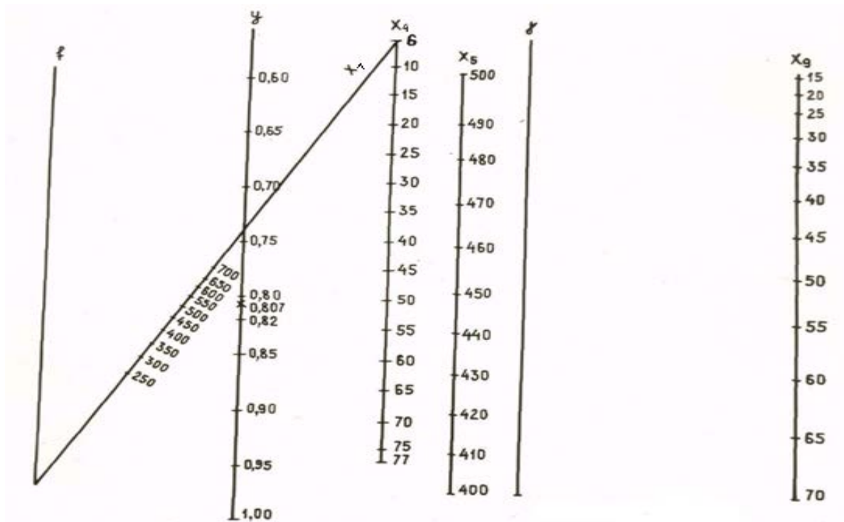
Рис. 2. Номограмма зависимости физиологического состояния ( y ) от тяжести работы X_7 , площади перекрытия усилительными накладками X_4 и воздухопроницаемости X_9 основной ткани спецодежды
