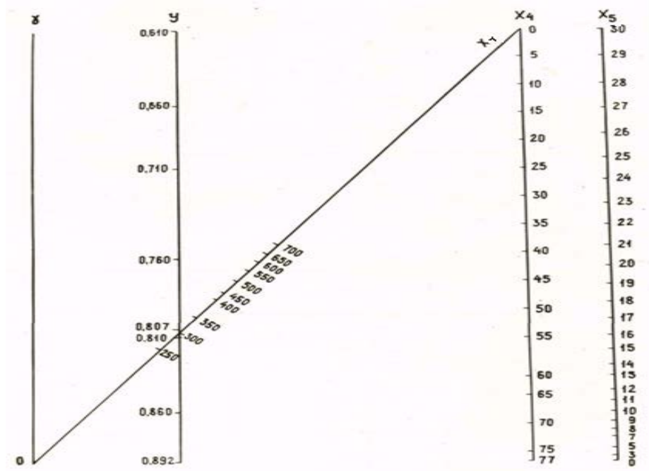
Рис. 1. Номограмма зависимости физиологического состояния горнорабочего ( y ) от тяжести работы X_7 , площади перекрытия усилительными накладками X_4 и содержанием синтетики (лавсана) в основной ткани X_5
