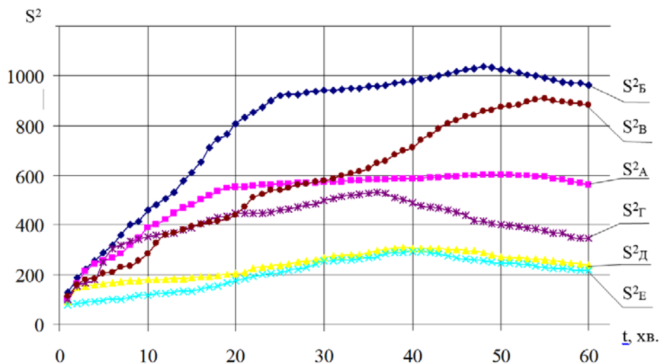
Рис.4. Дисперсія температур по обігрівальній поверхні несучої стіни під час обчислювального експерименту.
