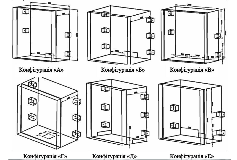
Рис.2. Конфігурації установок для проведення випробувань на вогнестійкість несучих стін.
