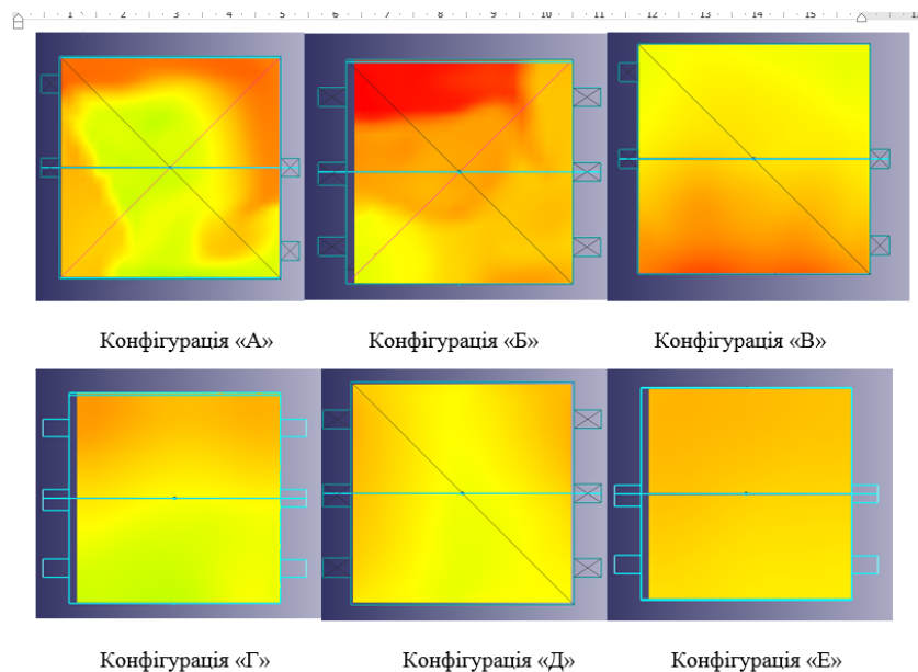
Рис.3. Градієнт температур по обігрівальній поверхні змодельованих конструкцій.
