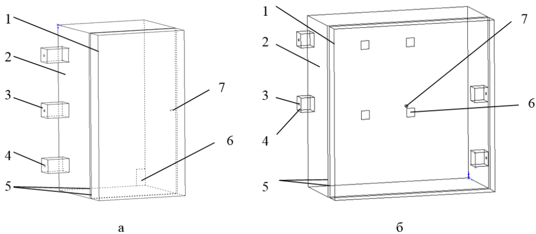
Рис. 1. Геометрична конфігурація вертикальних печей (а – Лабораторії 1 (зображено лише симетричну половину) та б – Лабораторії 2): 1 – огороження печі; 2 – фрагмент стіни; 3 – регіон вдуву; 4 – регіон форсунки; 5 – поверхні, що сполучаються; 6 – регіон виходу продуктів горіння; 7 – розрахункова область термопар.
