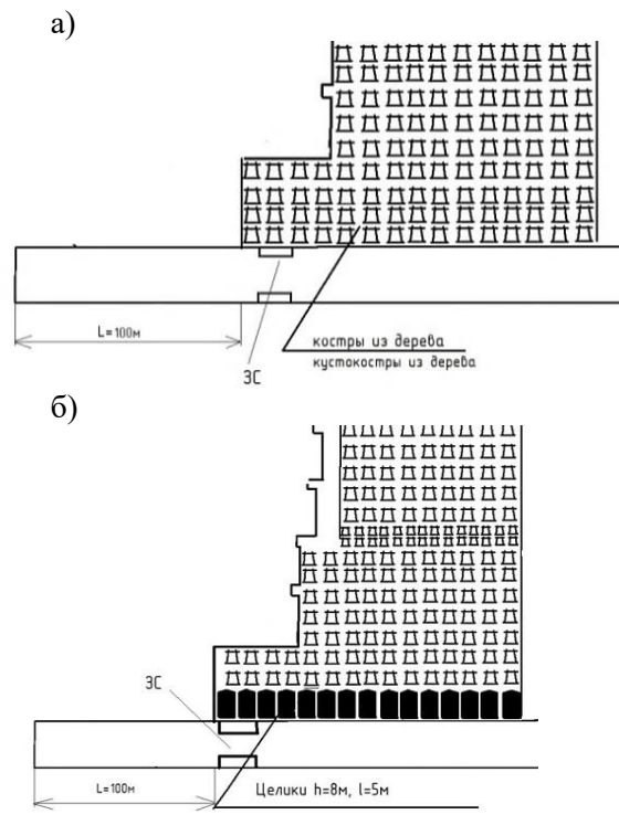
Рис. 1. Схема экспериментальных участков для определения смещений боковых пород на контуре откаточного штрека, пройденного по пласту I 3 «Мазурка», при охране (а) деревянными кострами или кустокострами, (б) целиками угля: ЗС – место расположения замерной станции.
