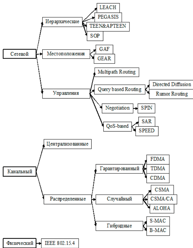
Рис. 1. Классификация основных протоколов передачи данных в WSN
