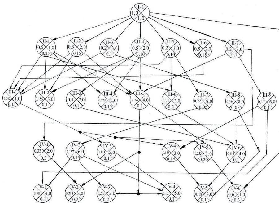
Рис. 6. Граф цілей дослідження (проекування) адаптивної АСКТП з елементами АСКВ електросталеплавильного агрегату за технологією «вищого рівня»
