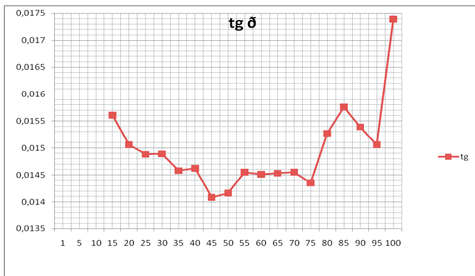
Рис. 1. Залежність tg δ від частоти для чистого латексу
