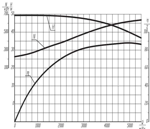
Рис. 2. Энергетические характеристики модернизированного насоса 24 НДС (с параметрами в рабочей точке Q = 5500 м³/ч, H = 38 м)
