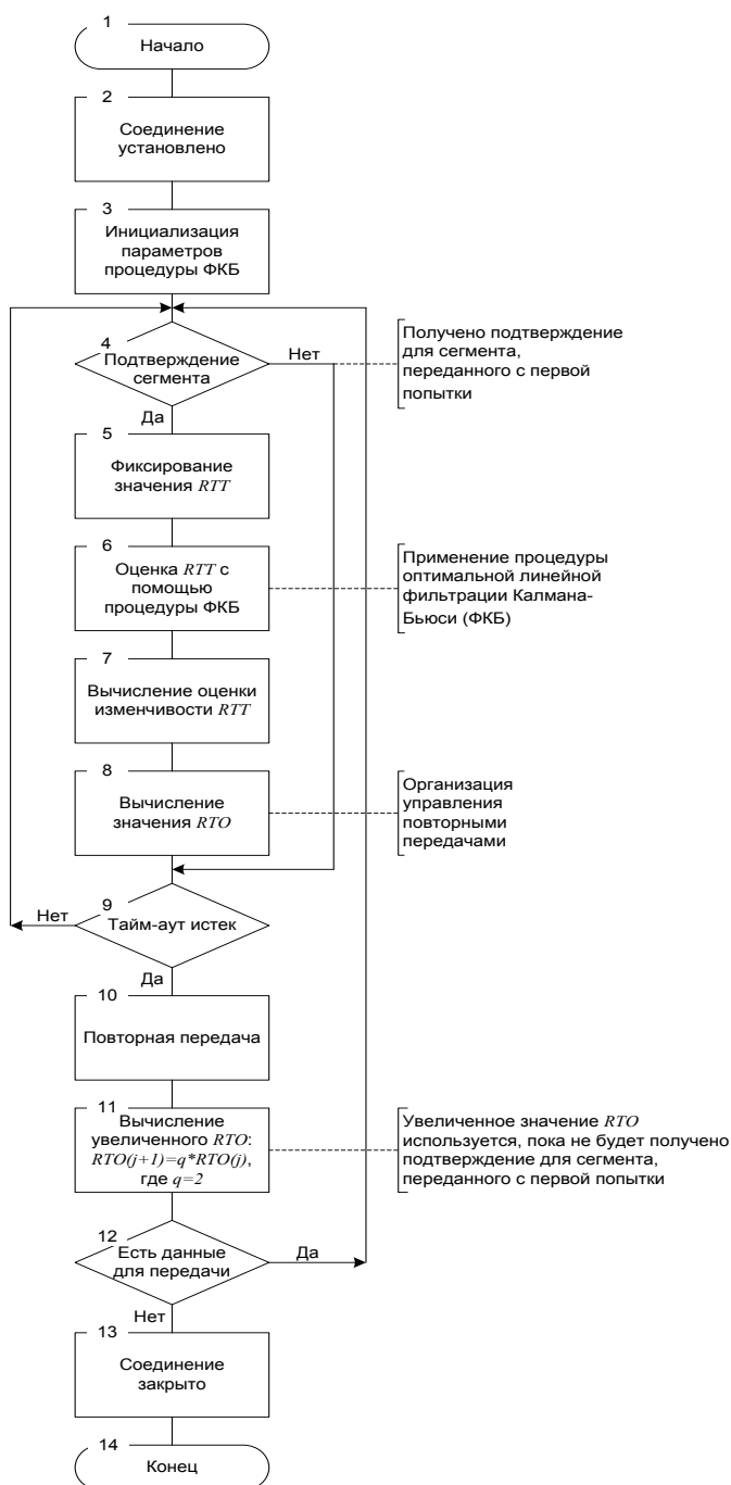
Рис.2. Структурная схема модернизированного метода вычисления RTO
