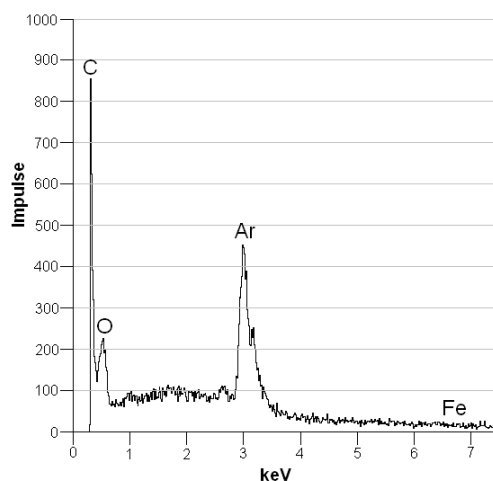
Рис. 5. Енергодисперсійний аналіз гідрогелю на основі ГЕМА-ПВП кополімеру, наповненого сріблом
