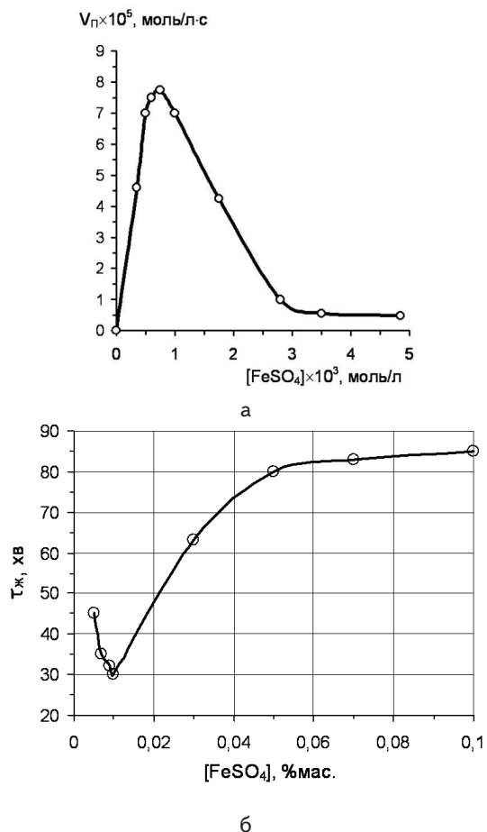
Рис. 2. Вплив концентрації \text{FeSO}_4 на кінетичні характеристики полімеризації: а - швидкість полімеризації V_p , моль/л·с (ГЕМА:ПВП: \text{H}_2\text{O} = 7:3:10 мас.ч.); б - час життєздатності композиції \tau_{ж} , хв (ГЕМА:ПВП: \text{H}_2\text{O} = 8:2:10 мас.ч.)
