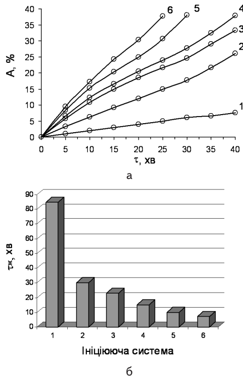
Рис. 3. Вплив складу ініціальної системи на кінетичні характеристики полімеризації: а - конверсія мономеру A , %; б - час життєздатності композиції \tau_{ж} , хв. [\text{FeSO}_4] = 0,01\% мас; \text{FeSO}_4:\text{In} = 1:1 ; T = 298 К
