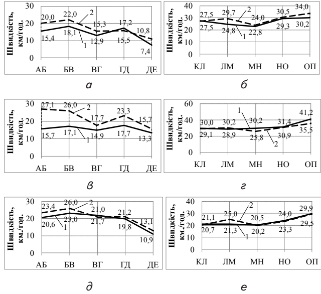
Рис. 1. Значення експлуатаційної швидкості руху автобуса: а, б, д – відповідно ранковий пік, непіковий період, вечірній пік для напрямку «до центру»; б, г, е – відповідно ранковий пік, непіковий період, вечірній пік для напрямку «від центру»; 1 – натурні дослідження; 2 – моделювання у VISUM
