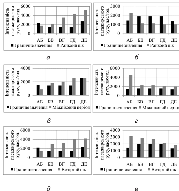
Рис. 2. Доцільність впровадження спеціальних смуг на перегонах вулиць за критерієм II: а, б, д – відповідно ранковий пік, непіковий період, вечірній пік для напрямку «до центру»; б, г, е – відповідно ранковий пік, непіковий період, вечірній пік для напрямку «від центру»
