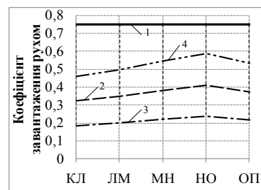
Рис. 4. Доцільність впровадження спеціальних смуг за критерієм III: а – до центру; б – від центру; 1 – верхня межа допустимої області завантаження на непріоритетних смугах; 2 – ранковий пік, 3 – непіковий період; 4 – вечірній пік
