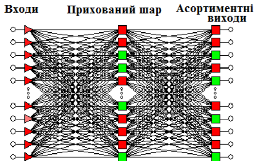
Рис. 3. Архітектура багатшарового перцептрона для задачі дослідження
