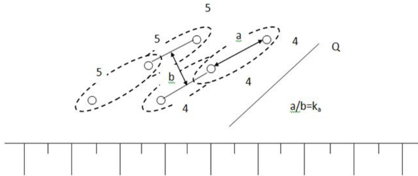
Рисунок 2 – Принципи розташування зарядів
