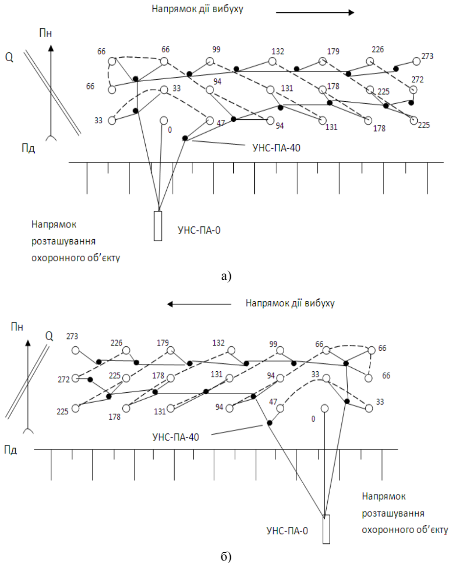
Рисунок 1 – Технологічна схема підривання відносно системи тріщинуватості Q: а) з лівим орієнтуванням врубу; б) з правим орієнтуванням врубу
