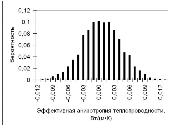
Рисунок 3 – Распределение вероятности реализации значений \delta\lambda_{ef}
