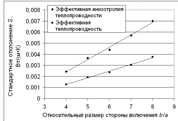
Рисунок 4 – Зависимость S_{at} и S_{tc} от размера включений
