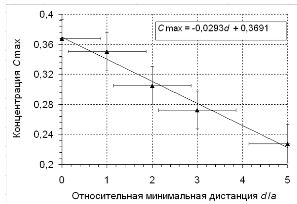
Рисунок 8 – Зависимость концентрации c_{max} для максимума S_{tc} от минимальной дистанции d
