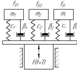
Рисунок 1 – Розрахункова схема багатомасового ВО
