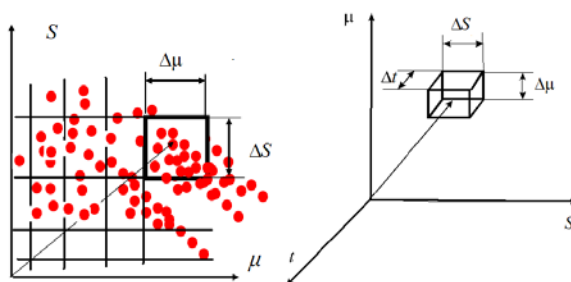
Рис. 2. Элементарная ячейка фазового технологического пространства
