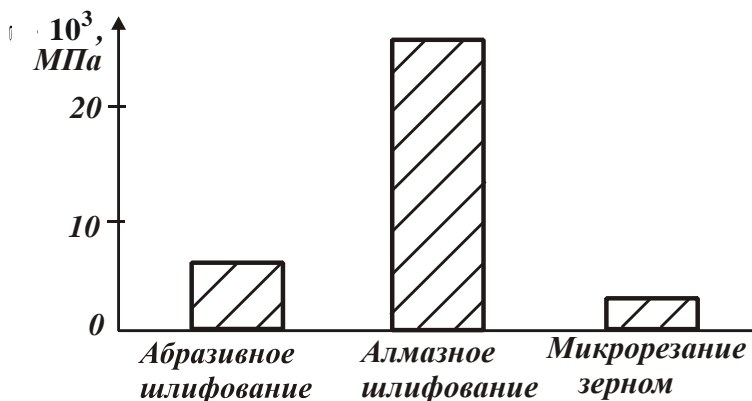
Рис. 8. Значения энергоемкости обработки \sigma для разных условий обработки.
