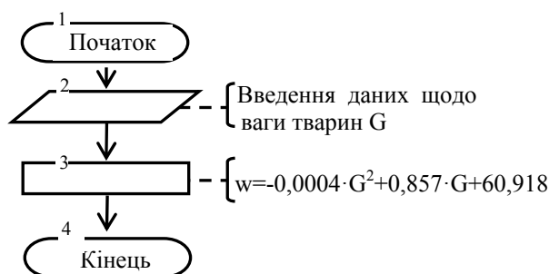
Рисунок 3 - Блок-схема алгоритму визначення за виразом (1) кількості виділення вологи однією твариною молодняку ВРХ віком від 6 місяців при температурі навколишнього середовища +10 °С
