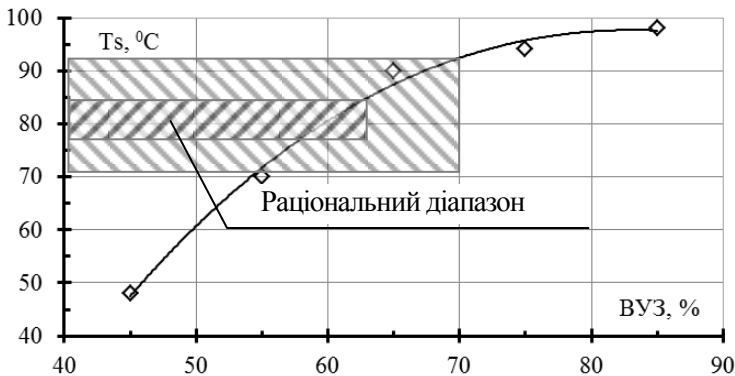
Рис. 4. Залежність термічної стійкості білкової основи від ВУЗ
